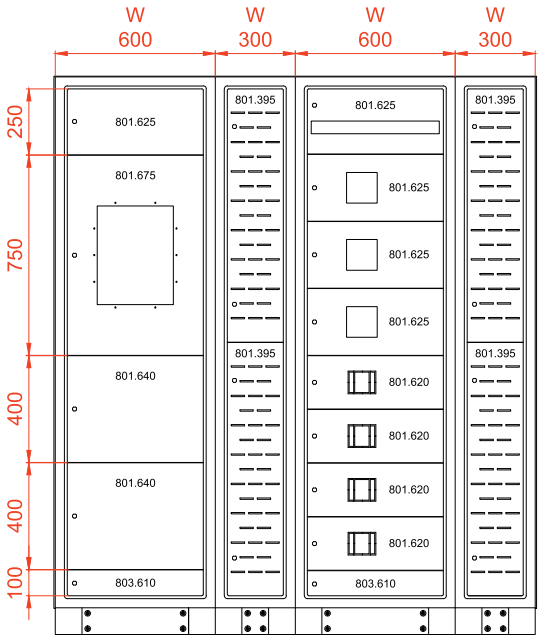
Placas de cubierta interiores
