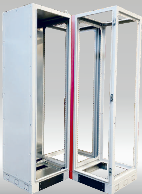
RIEL DE MODULO DE ESQUINA (ANCHO 50 mm)
